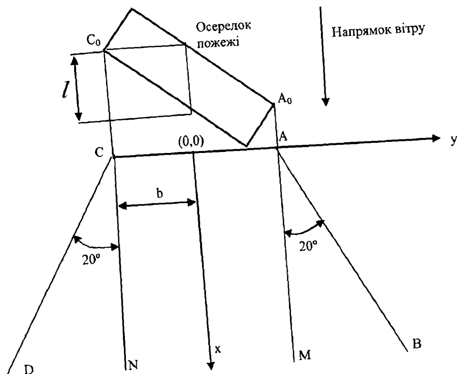
Рисунок 4 – Схема визначення розмірів зон загазованості від окремого осередку пожежі при напрямку вітру під гострим кутом до фасаду будівлі
