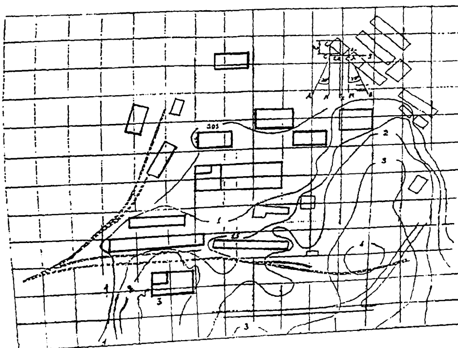
Рисунок 5 – Схема визначення розмірів зон загазованості для різних осередків пожежі
